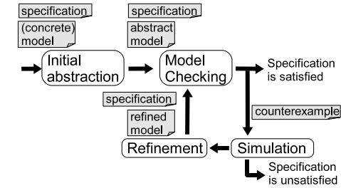
図 1 一般的な CEGAR アルゴリズム
