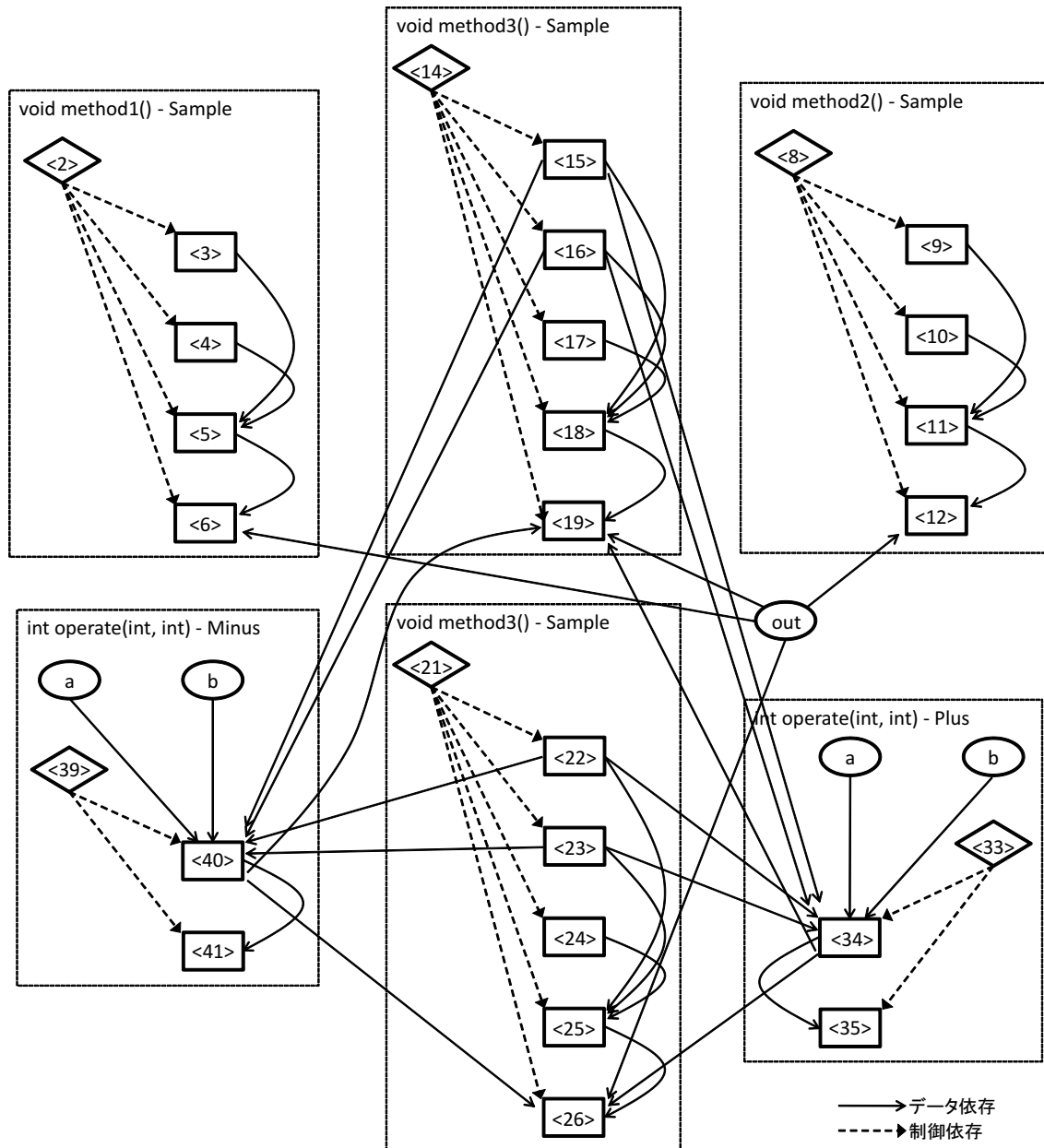
図 2 サンプルソースコードから生成された SDG
