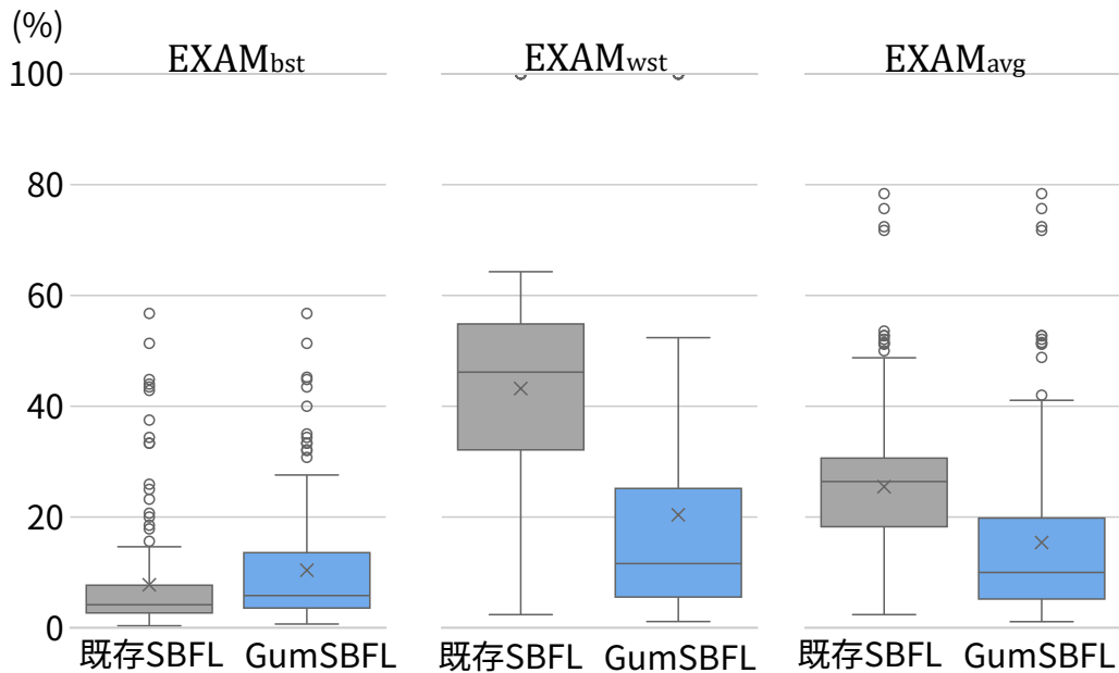
図 3 欠陥限局精度の比較
