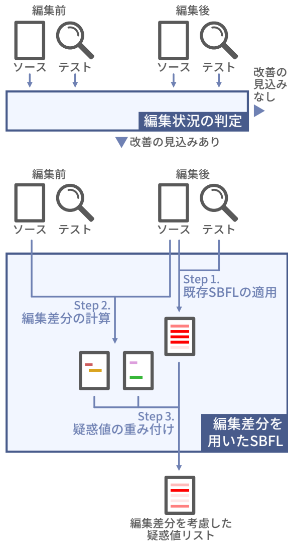
図 2 提案手法の概要図
