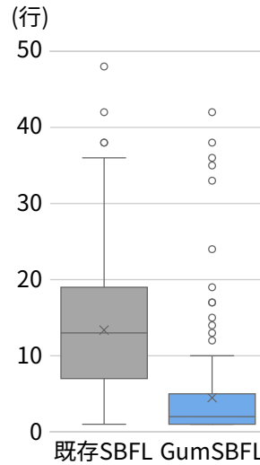
図5 欠陥行と同順位の行数の分布
