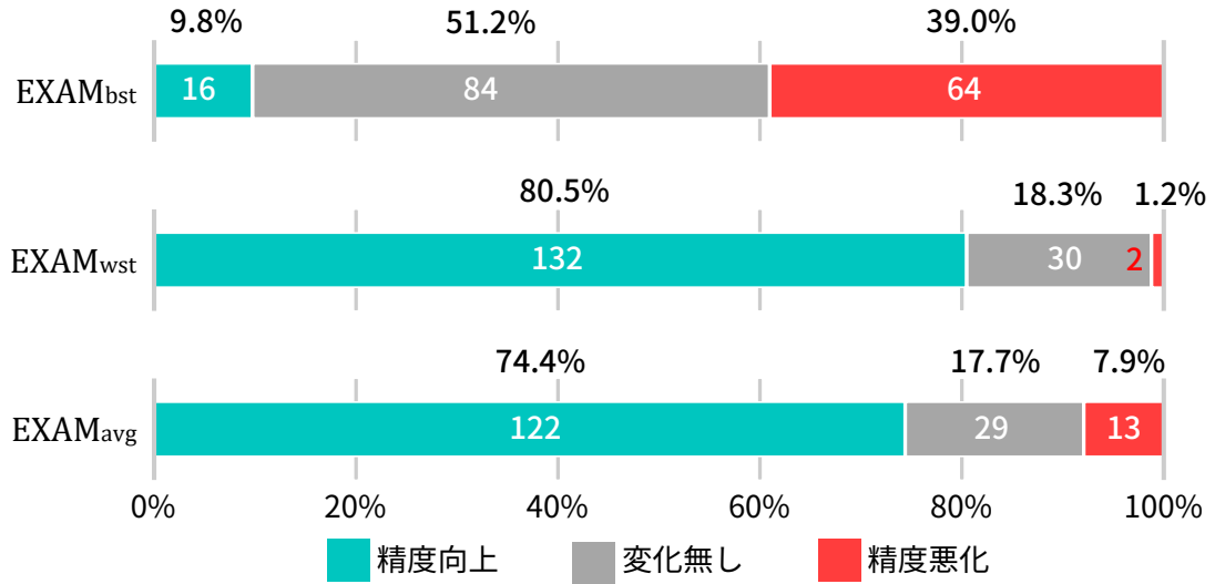
図4 EXAM が変化した事例の割合
