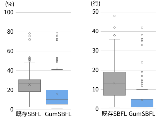
図 3: 欠陥限局精度の比較 図 4: 欠陥行と同じ疑惑値をもつ行数の比較
