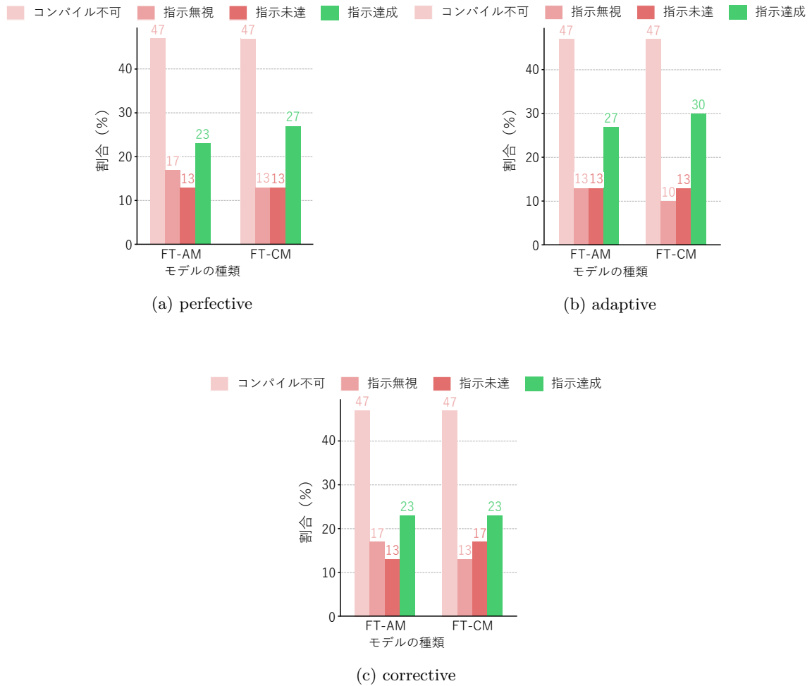
図 3: 改変指示の具象度と改変後ソースコードの割合
