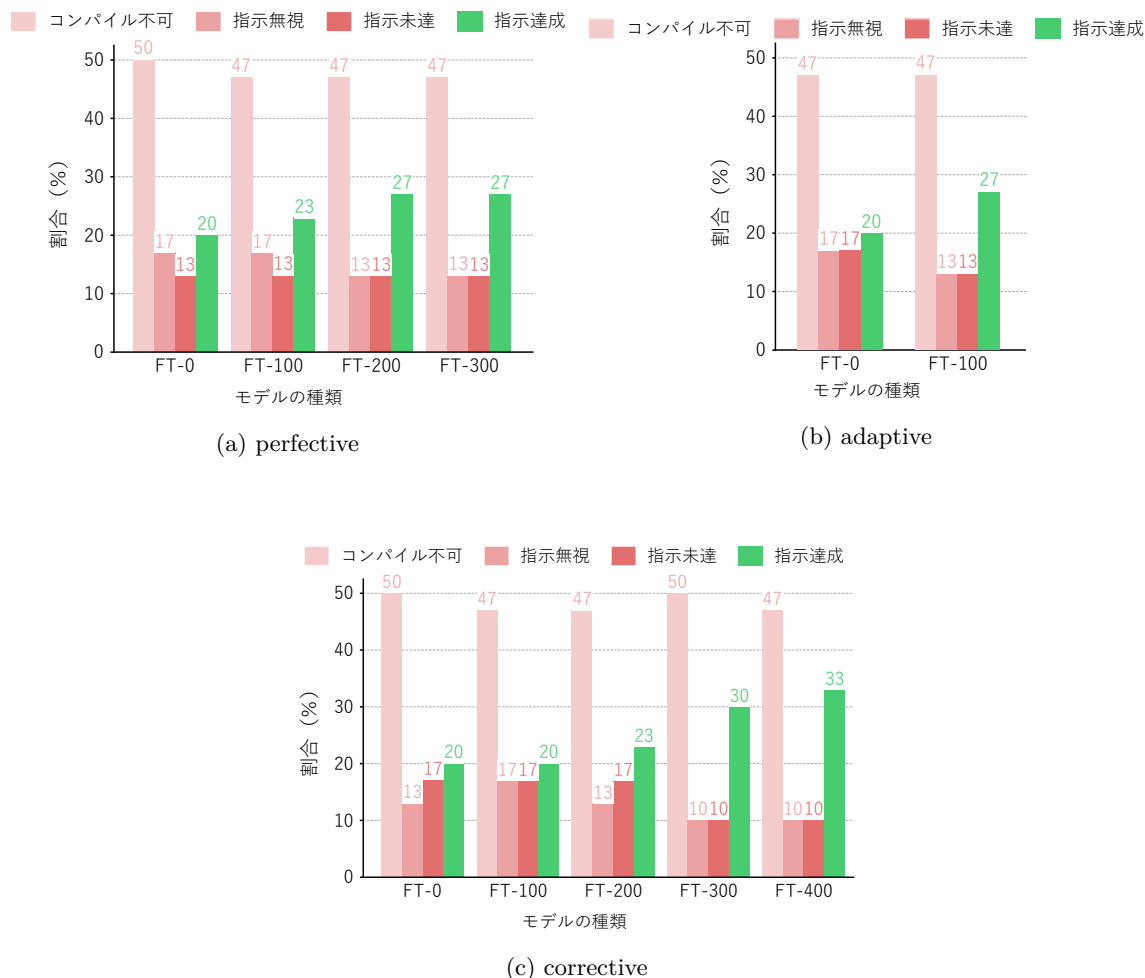
図 2: 再学習データセットの量と改変後ソースコードの割合
