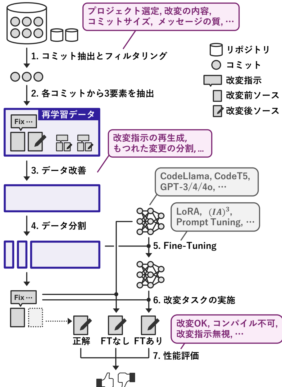
図 1: 実験の流れ
