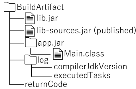
図 5: BuildArtifact が保持する成果物例
