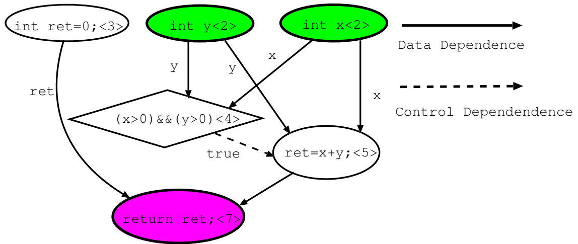
図 7: PDG の例
