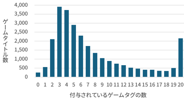
図3 データセットの1ゲーム当たりのタグ数の分布
