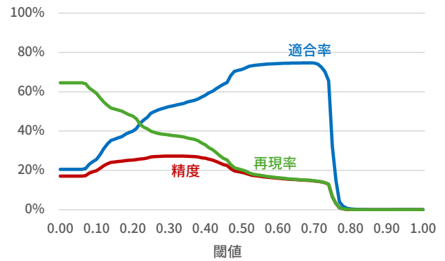
図5 閾値ごとのタグ予測性能
