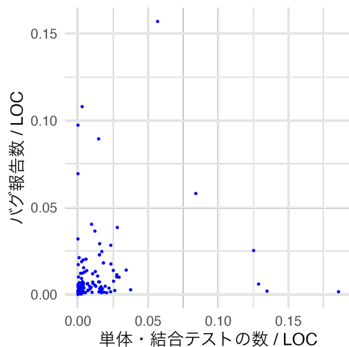
(a) (バグ報告数 / LOC) と (単体・結合テストのテストケース数 / LOC) との間の相関を表す散布図
