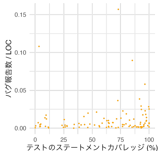
(b) (バグ報告数 / LOC) と単体・結合テストのステートメントカバレッジとの間の相関を表す散布図
