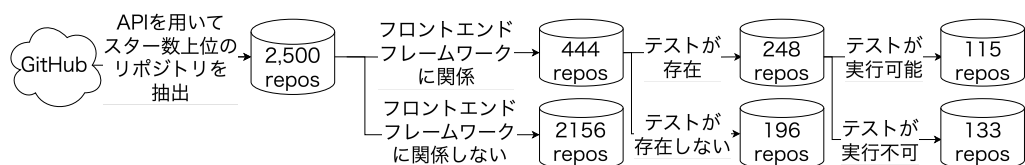
図 2: リポジトリをフィルタリングする詳細なフロー
