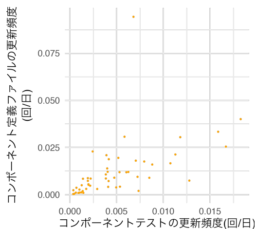
(b) コンポーネントテストの更新頻度とコンポーネント定義ファイルの更新頻度との相関を表す図
