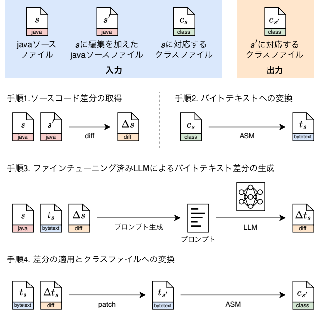
図 2: 提案手法の流れ
