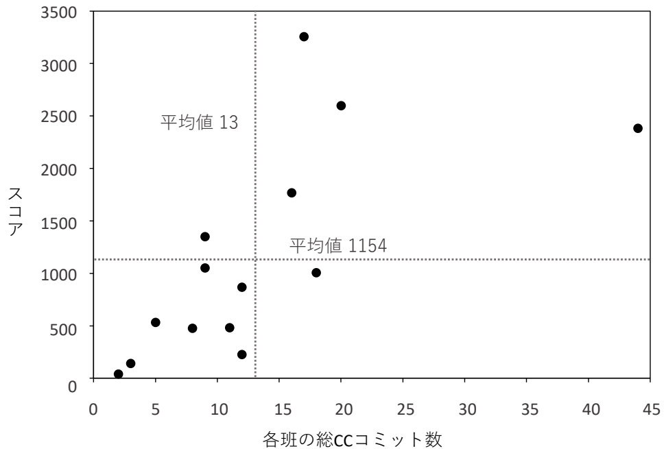
図7 各班の総 CC コミット数と対戦スコアの散布図
