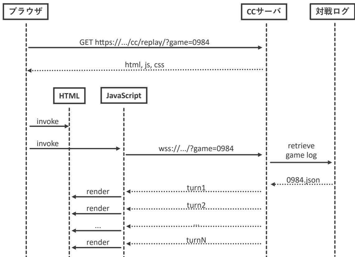
図 4 リプレイ機能のシーケンス図
