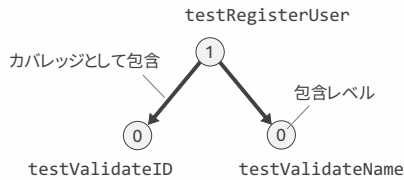
図3 包含グラフの例
