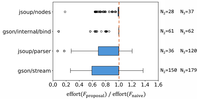
図6 ORD：naiveのデバッグ労力値に対するproposalのそのの比
