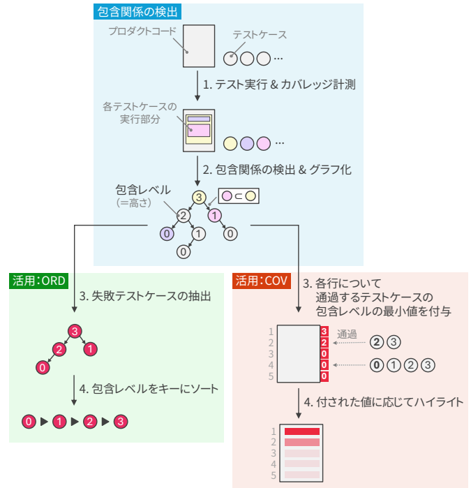
図4 2つの活用 (ORD と COV) の流れ
