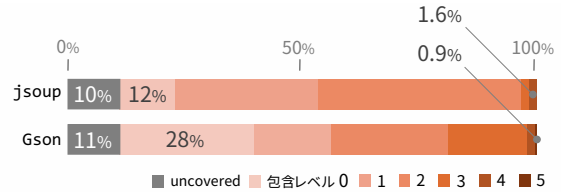
図7 COV：プロダクトコードの全行に対する包含レベルの内訳
