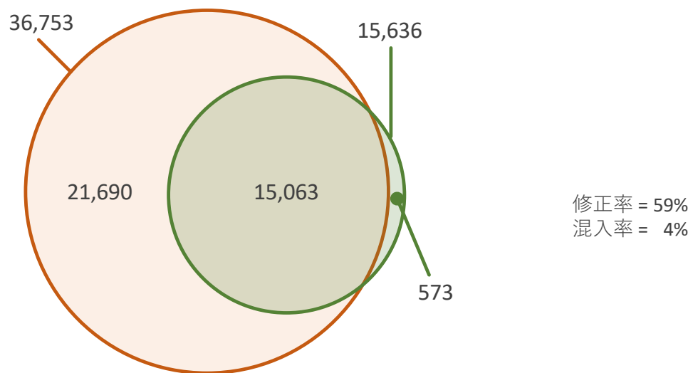
図7 識別子歪みのベン図 (Fernflower)
