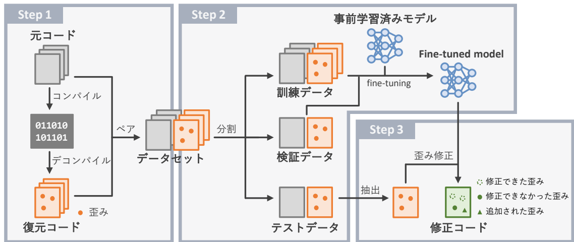
図2 提案手法による歪み修正の流れ
