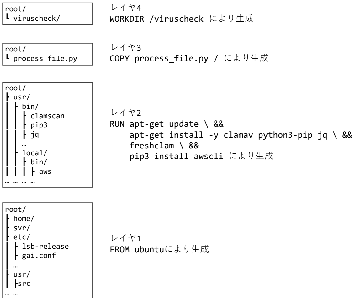
図 2: 図 1 の Dockerfile により構築される Docker イメージ
