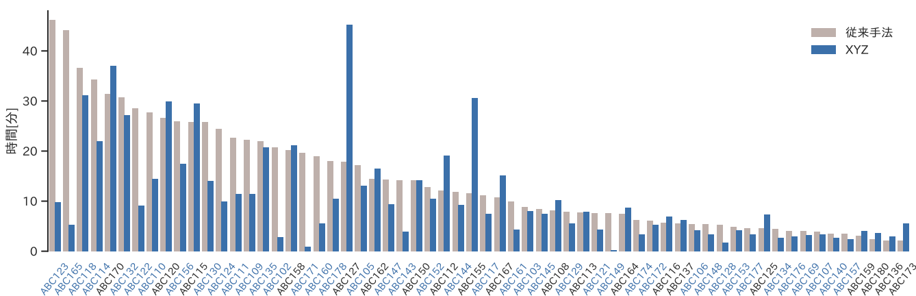
図 7 各問題に対する生成時間の比較
