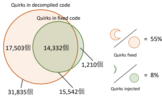
図 5: 識別子歪みのベン図
