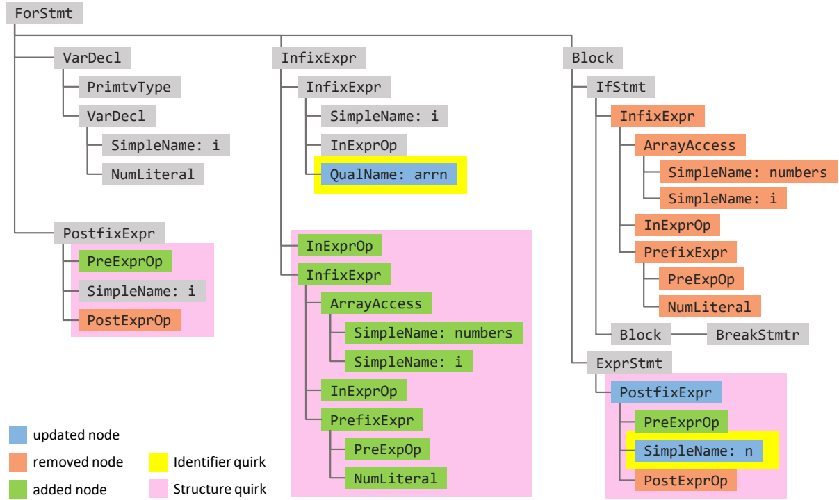
図 3: GumTree を用いた歪み検出の例
