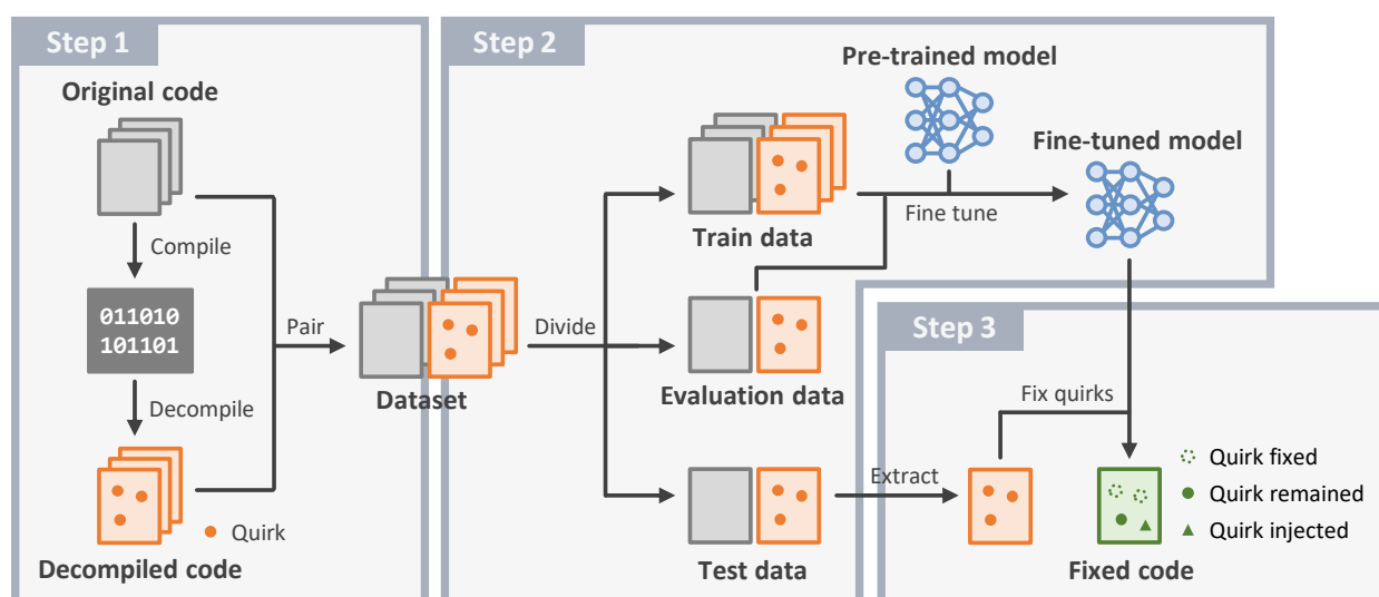
図 2: 提案手法による歪み修正の流れ
