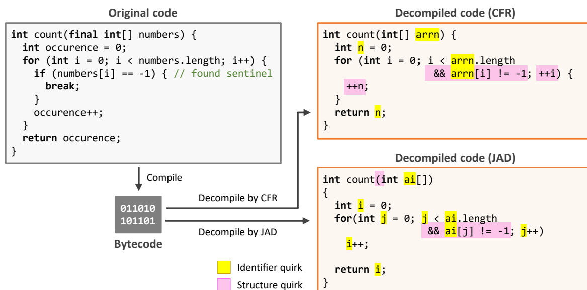
図 1: デコンパイラによって発生した歪みの例
