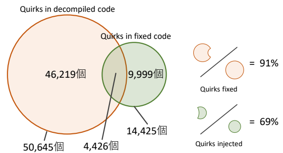
図 6: 構造的歪みのベン図
