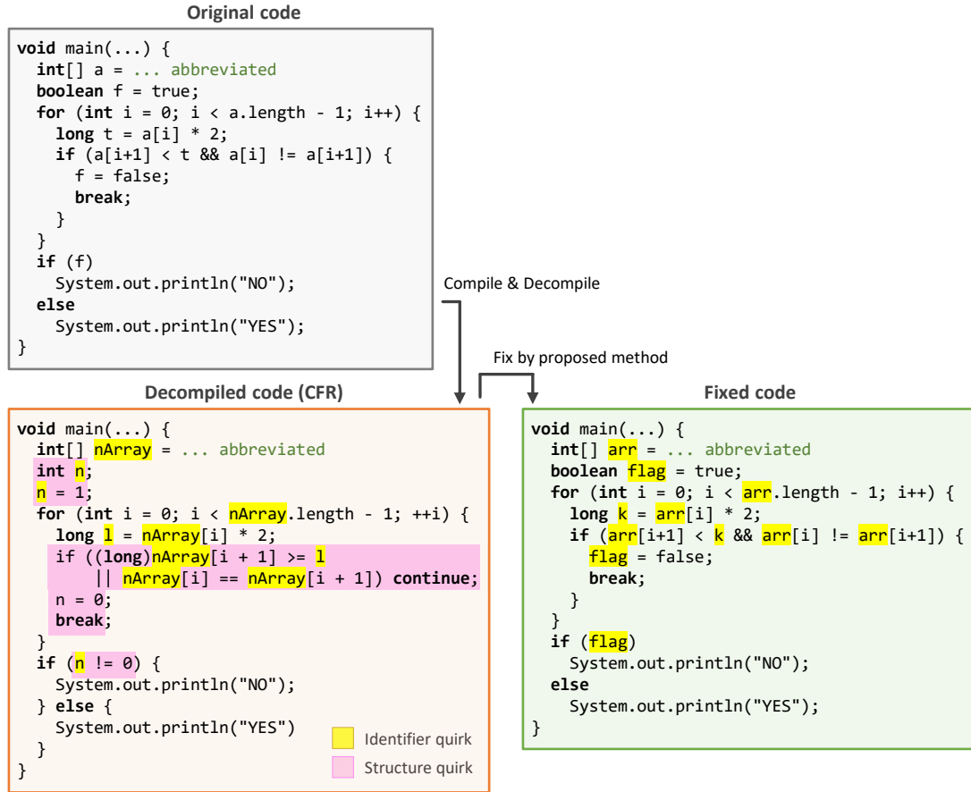
図 7: ReCa のある題材における歪み修正の実例
