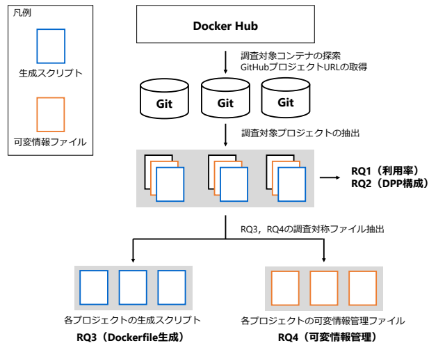
図5 調査全体の流れ
