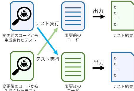
図 2: 交差実行の概要
