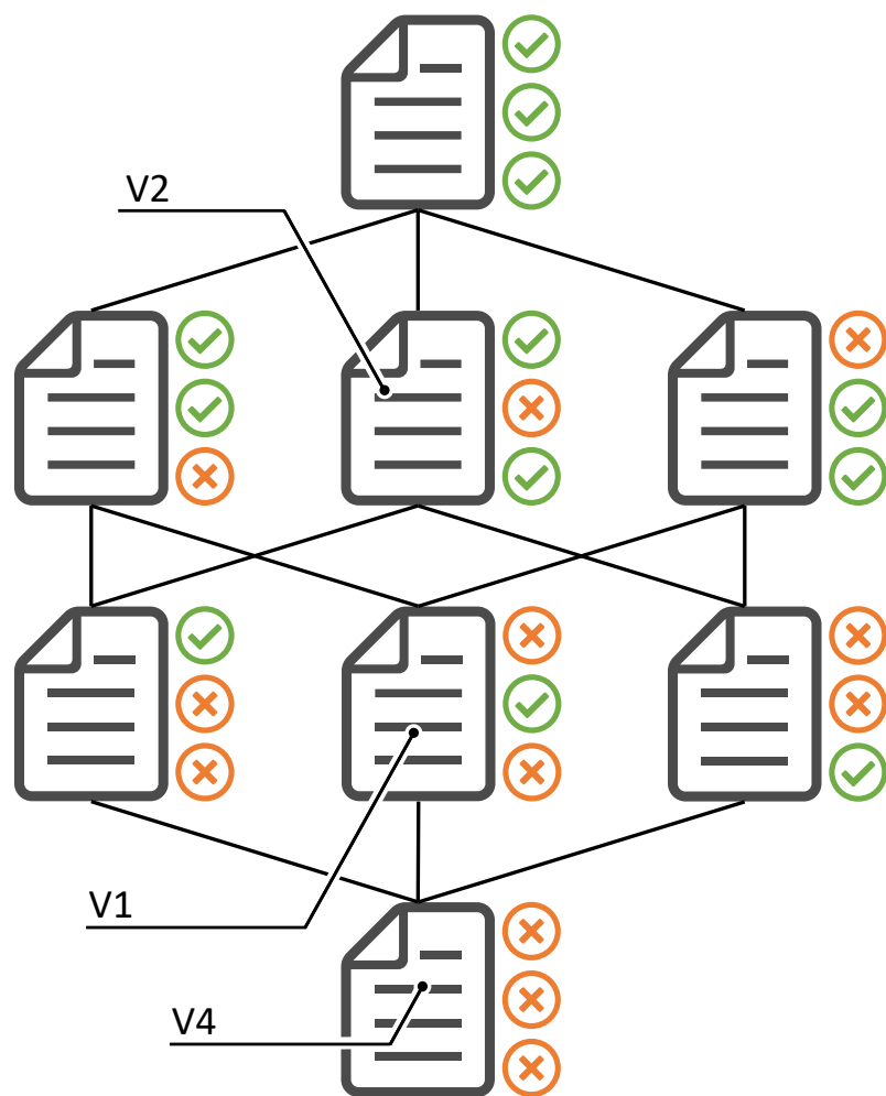
図4 テスト数3のときの全個体の関係
