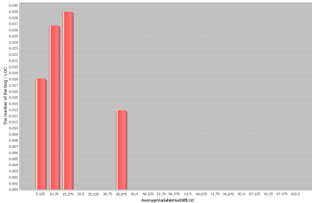
(b) 1 行あたりのバグ数
