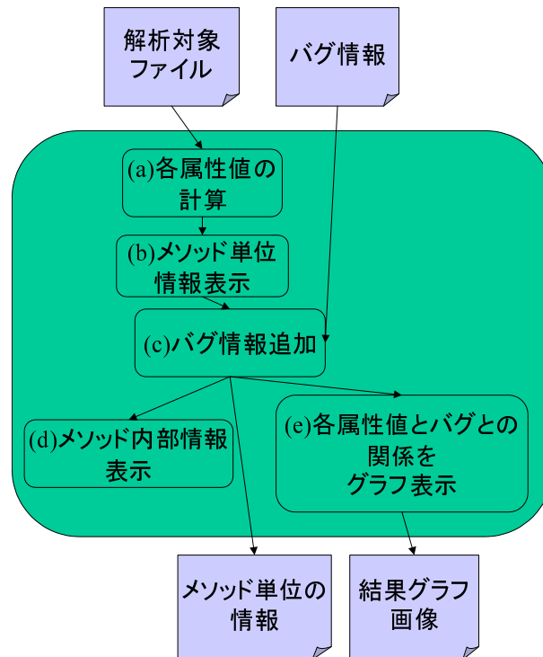
図 2: ツールの処理の流れ
