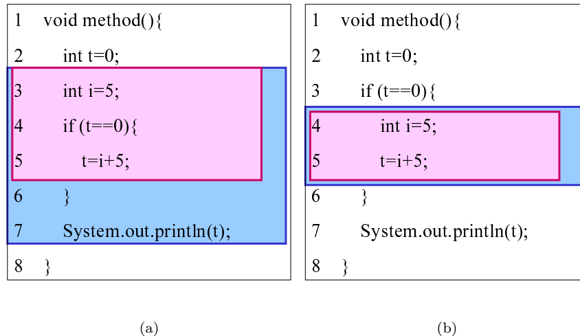
図 1: 変数のスコープと実際に使用されている範囲の例 青は変数のスコープを表し、赤は実際に使用されている範囲を表す
