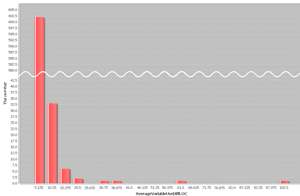
(a) メソッド数
