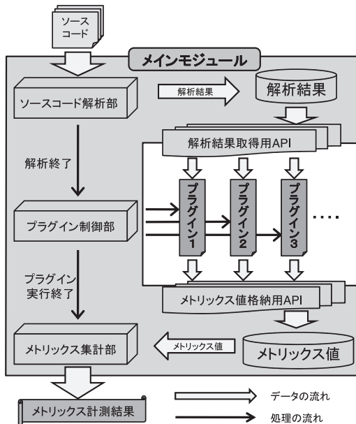
図 1 MASU の構成図
