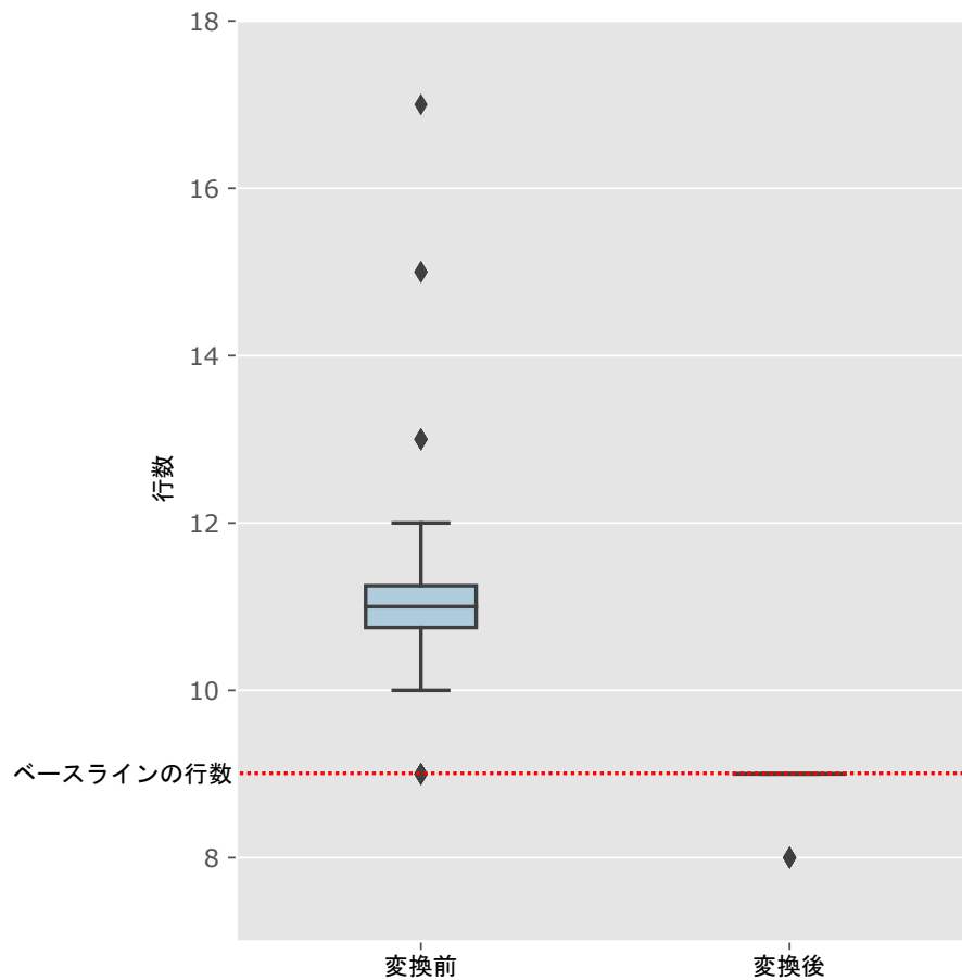
図 8: 変換前後での行数の比較
