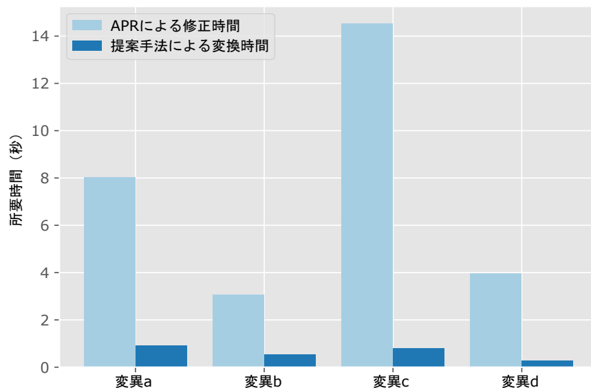
図 11: 修正と変換の所要時間の比較
