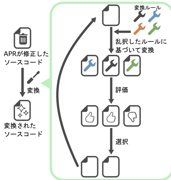
図 2: 提案する探索的変換手法の概要
