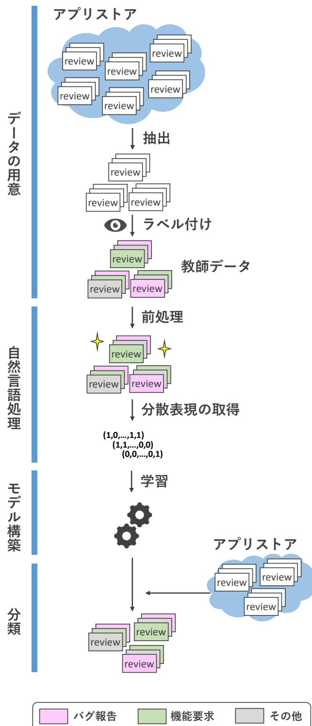
図1 既存手法の流れ
