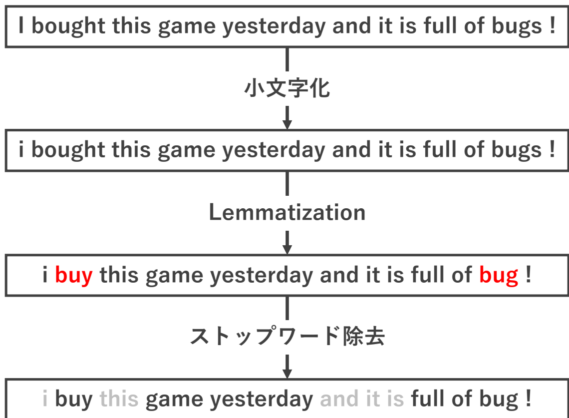
図 5 自然言語処理の流れ
