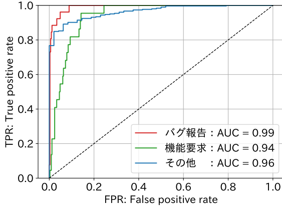
(a) E(R_{\text{Cities}} \Rightarrow R_{\text{Cities}}) の ROC 曲線
