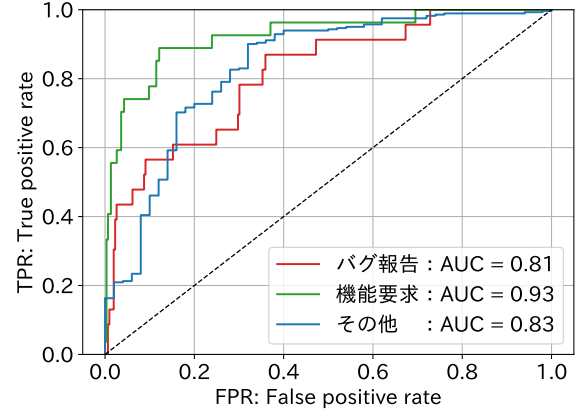
(e) E(F_{\text{Euro}} \Rightarrow R_{\text{Euro}}) の ROC 曲線
