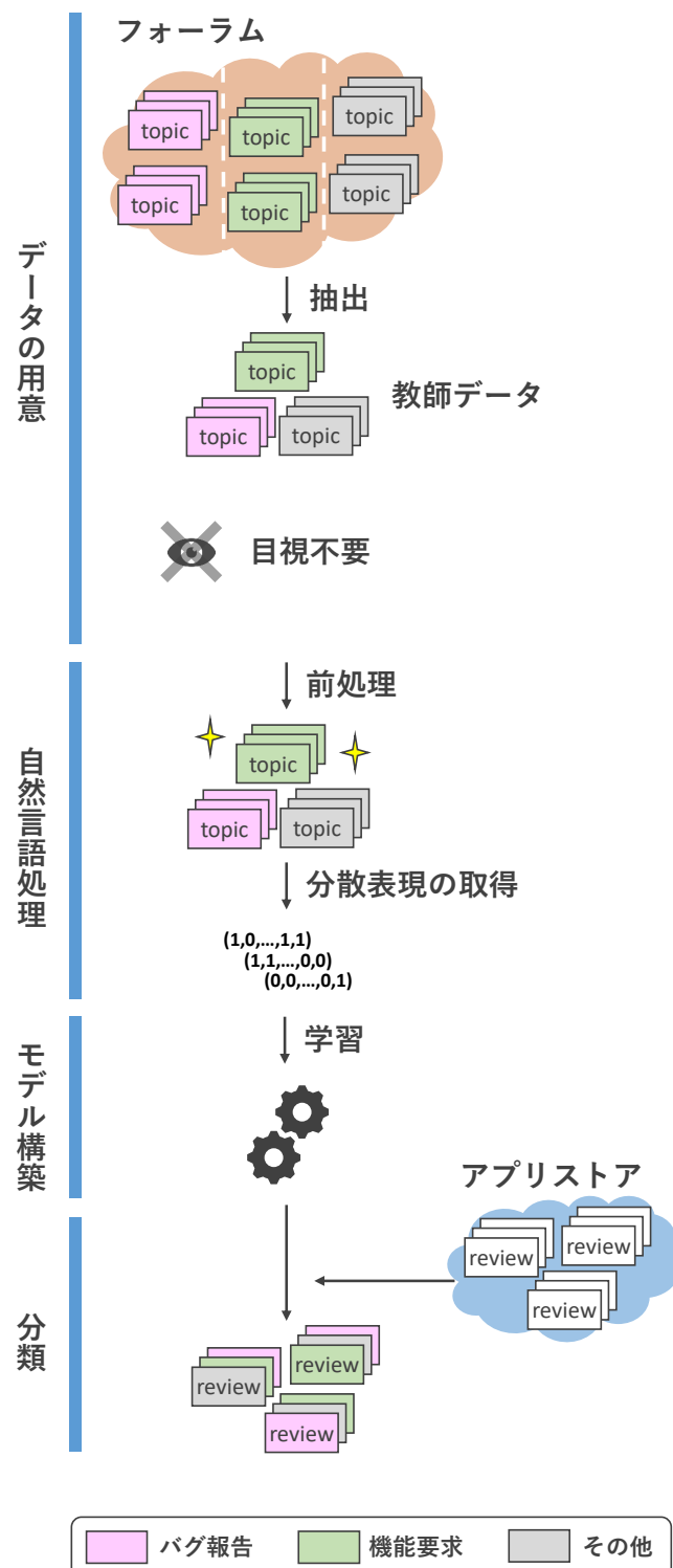
図4 提案手法の流れ
