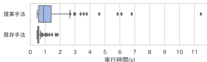
図 9 それぞれの手法による実行時間の比較
