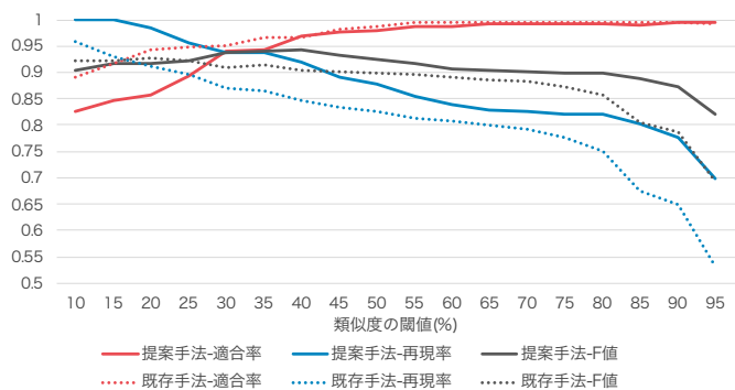
図6 手法別による適合率・再現率・F値
