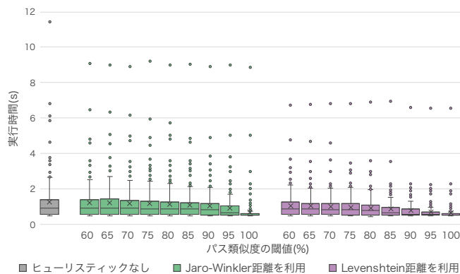
図 10 ヒューリスティックを利用した場合の実行時間の比較
