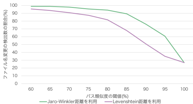
図 11 ヒューリスティック適用時に検出するファイル名の変更数の割合
