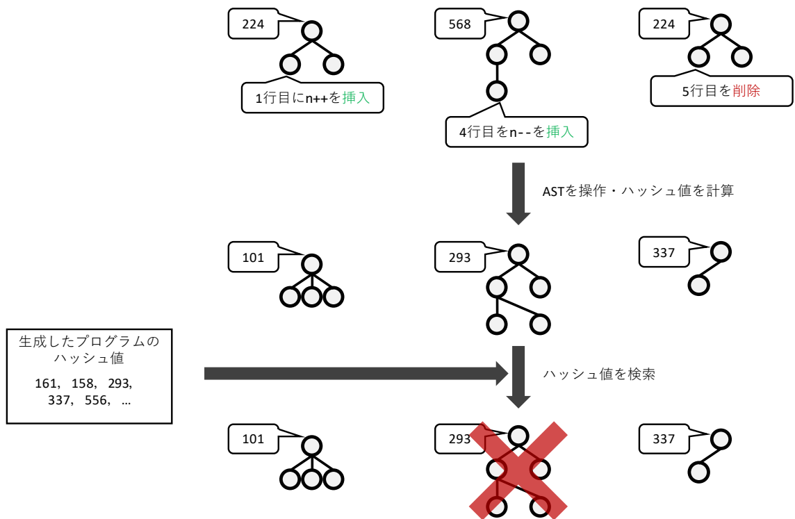
図 10 kGenProg の重複排除処理
