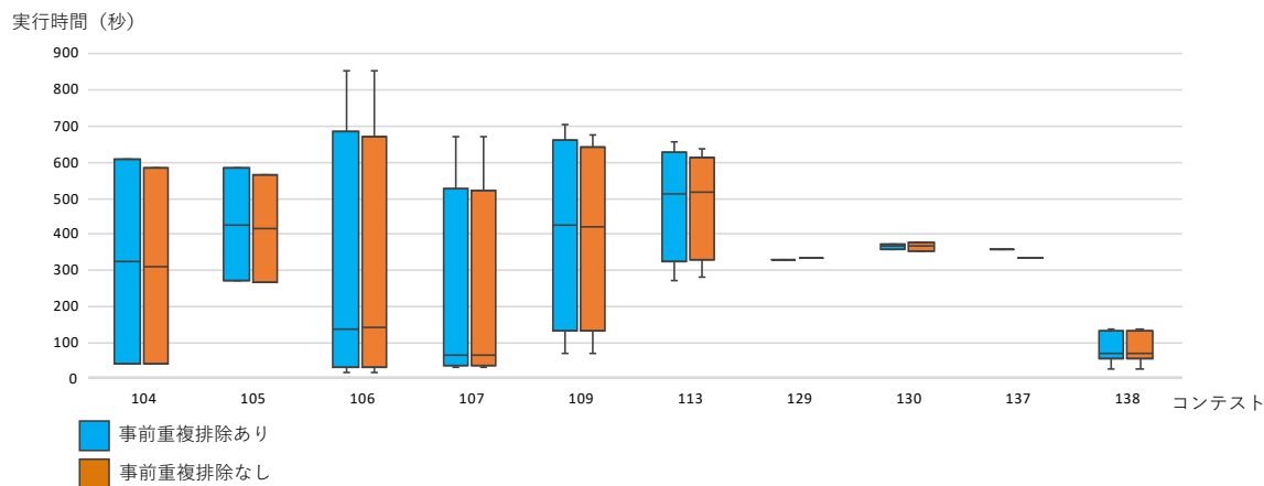
図 16 実行時間
