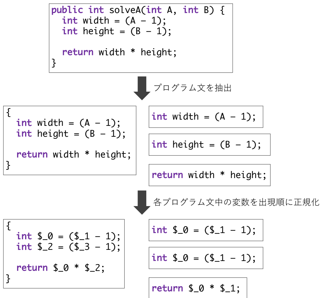
図4 変数の正規化の流れ
