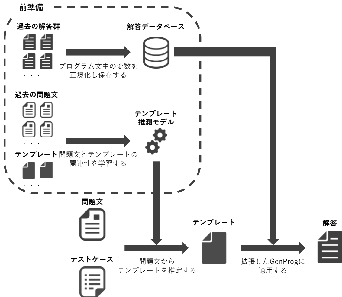
図6 手法の流れ
