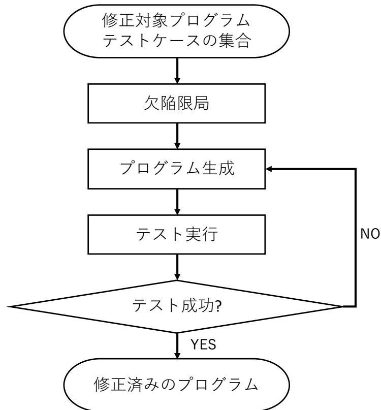
図1 GenProg の流れ
