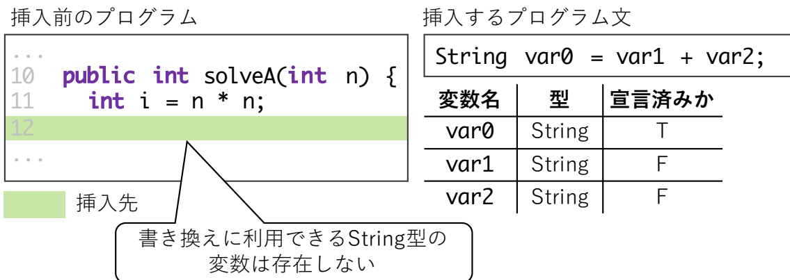
図 14 変数の書き換えの失敗例
