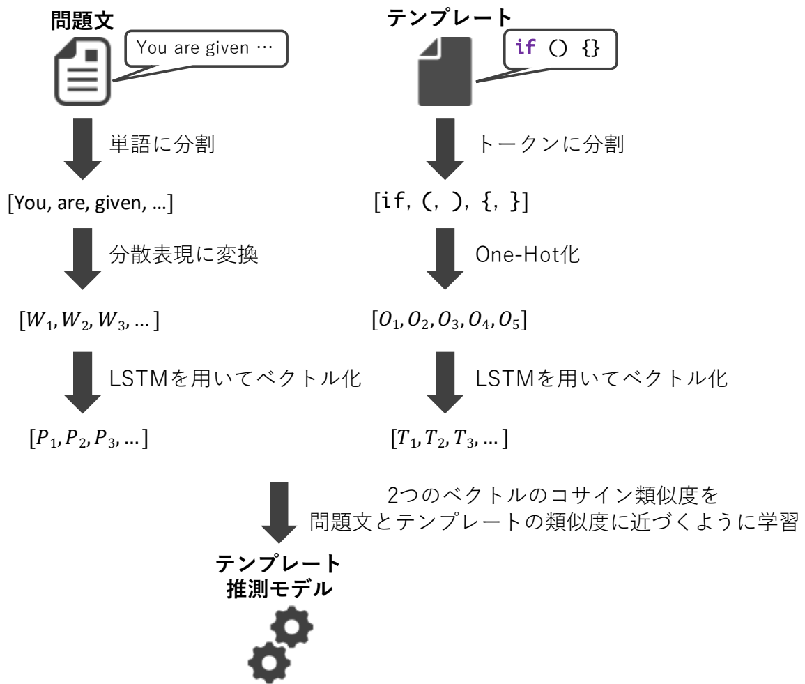
図8 テンプレート学習部の流れ
