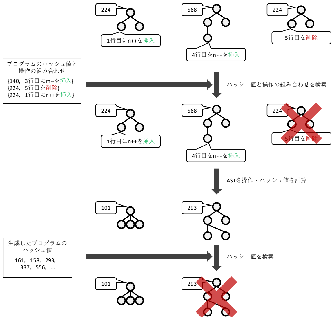
図 11 提案手法の重複排除処理
