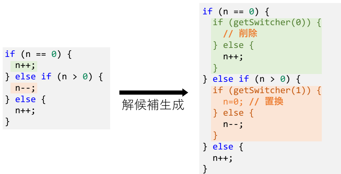
図 3 提案手法のコード生成
