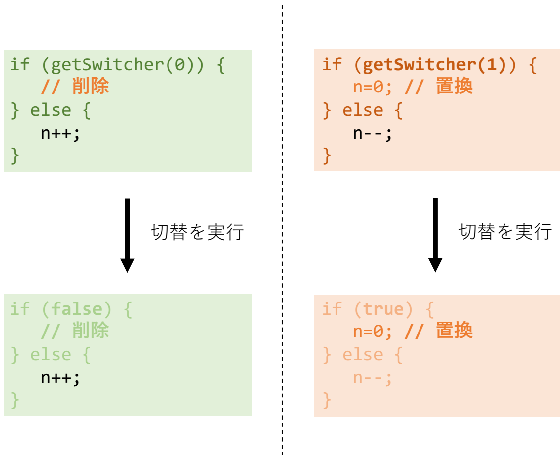
図 6 動的切替が実行されたプログラム
