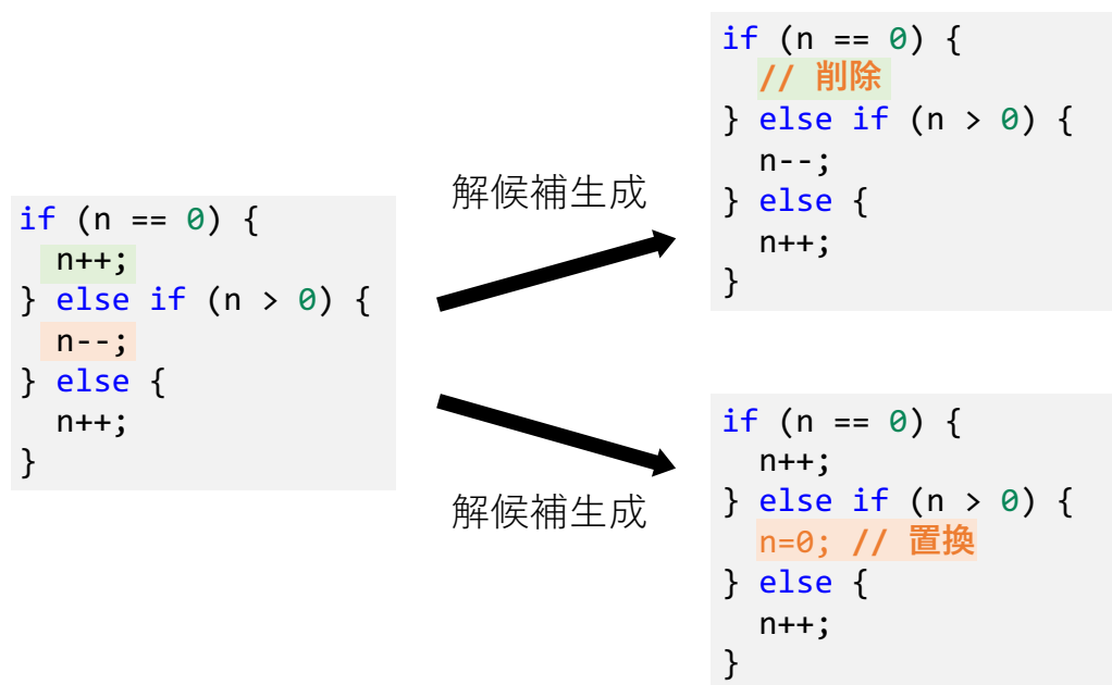
図2 従来手法のコード生成
