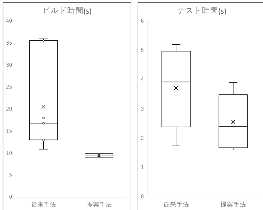
図 13 Apache Commons Math の実行結果
