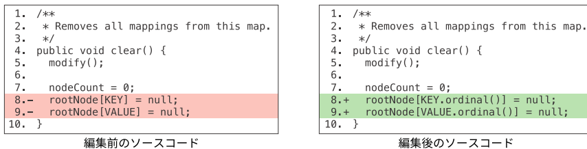
図 6 図 2 のソースコードに対して diff を実行した結果
