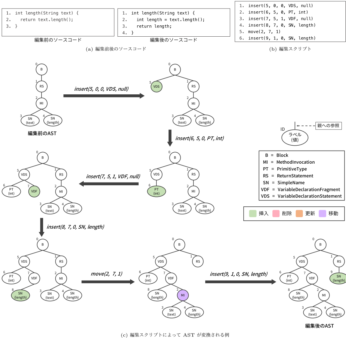
図 1 編集スクリプトの例と，その編集スクリプトに基づいて AST を操作する例 Fig.1 An example of an edit script, and an example that it converts AST.
