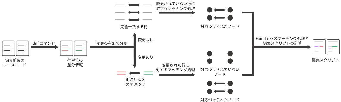
図 4 提案手法の概要
