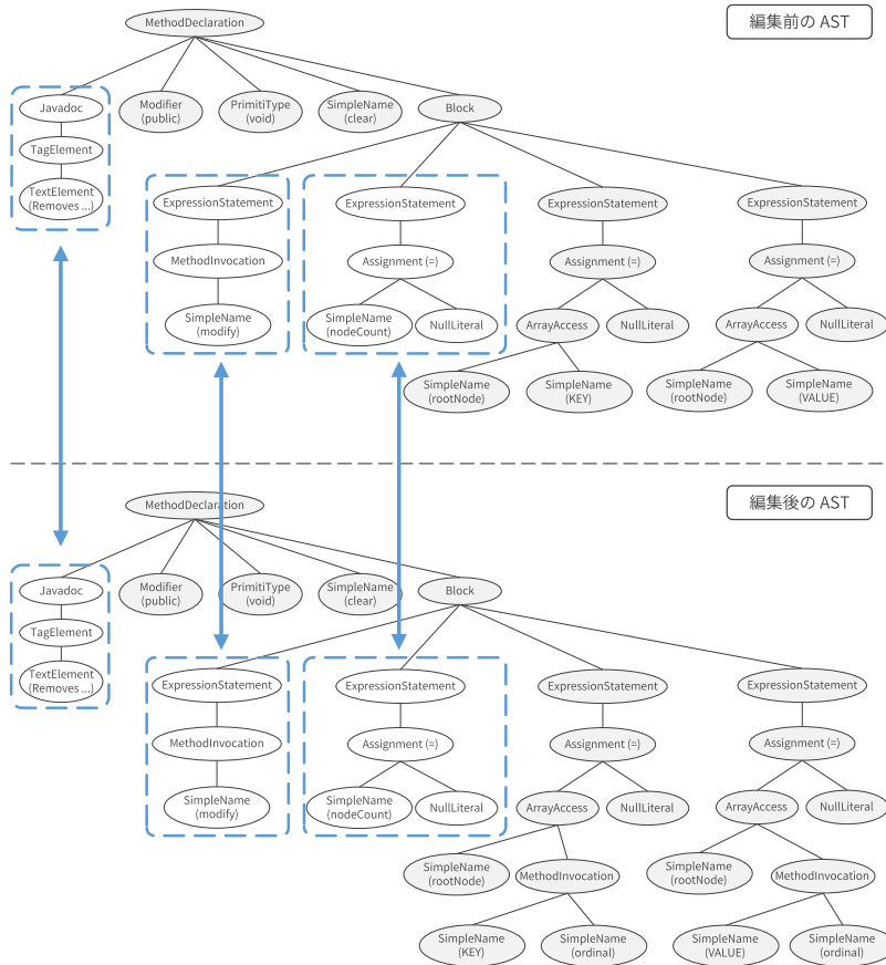
図 3 マッチング処理の結果. 白色のノードは対応づけられたノードを, 灰色のノードは対応づけられなかったノードを表している. 図を簡潔にするため, この図では部分木単位での対応づけのみ示しているが, 実際は各ノードが 1 対 1 で対応づけられている.
