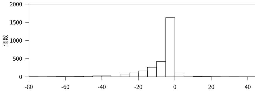
提案手法が出力する編集スクリプトの長さからGumTreeが出力する編集スクリプトの長さを引いた値
