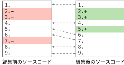
図 7 行単位の差分の例。破線は変更のない行の対応関係を表している。
