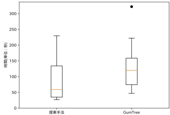
図 9 各差分を理解するのに費やした時間の中央値の箱ひげ図
