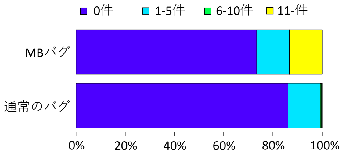
図 3 RQ1a: 重複報告件数
