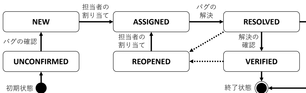
図2 BMO のバグライフサイクル
