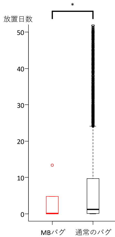
図 6 RQ2b: 放置期間
