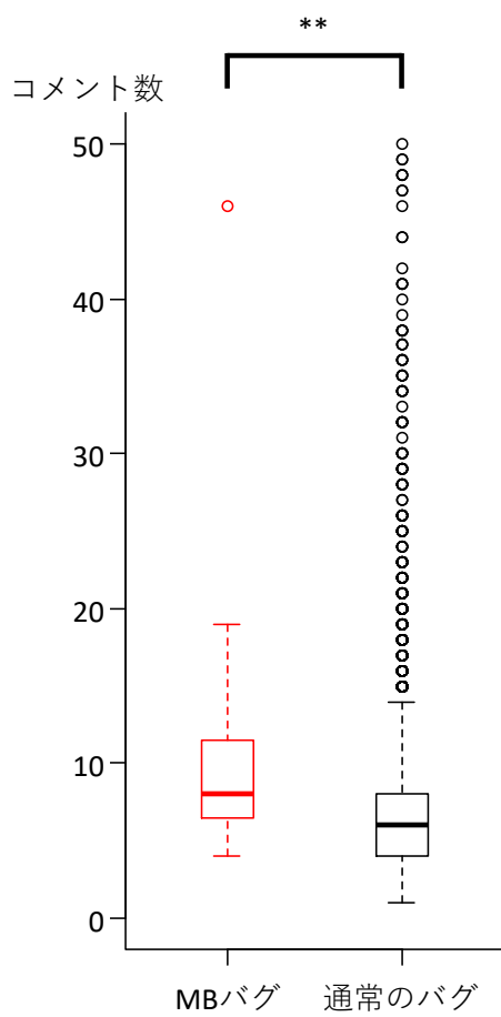
図7 RQ2c: コメント数
