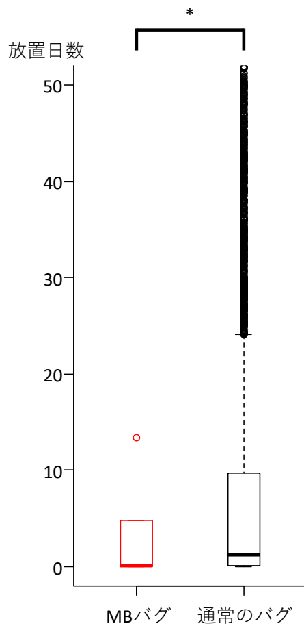
図 5 RQ2a: 修正期間
