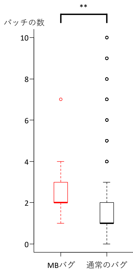
図8 RQ2d: 修正パッチの提案回数
