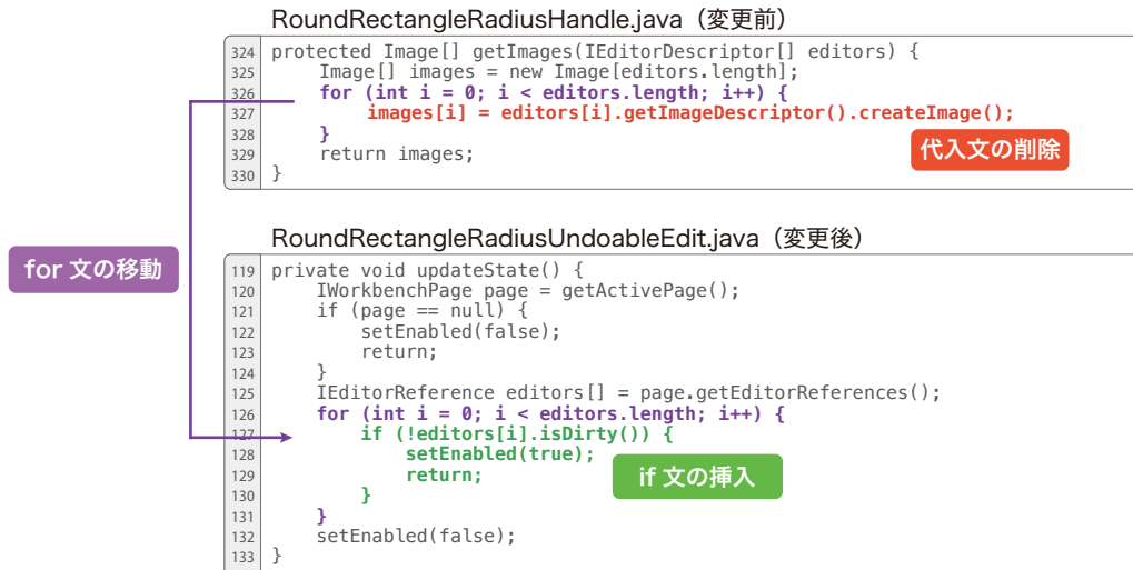
図 8 移動元と移動先のソースコードが大きく異なる例
