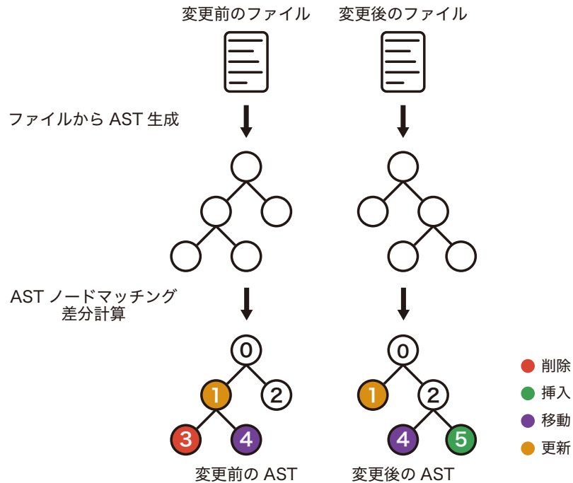
図 1 GumTree の差分検出
