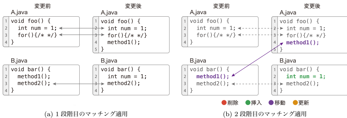
図 7 2段階のマッチングを適用した際の出力
