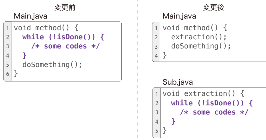
図 12 メソッドへの切り出しのソースコードの例
