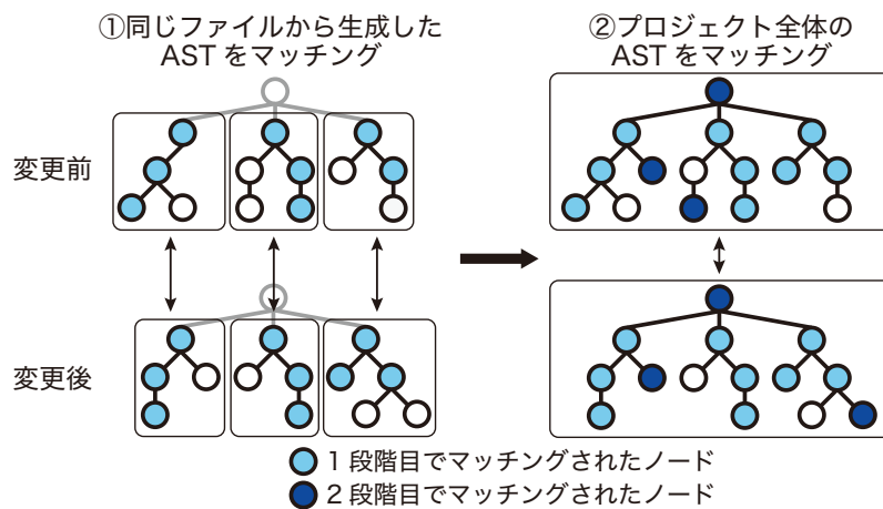
図6 2段階のマッチング
