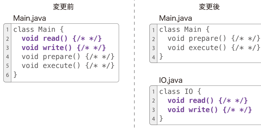
図 11 機能の分割のソースコードの例
