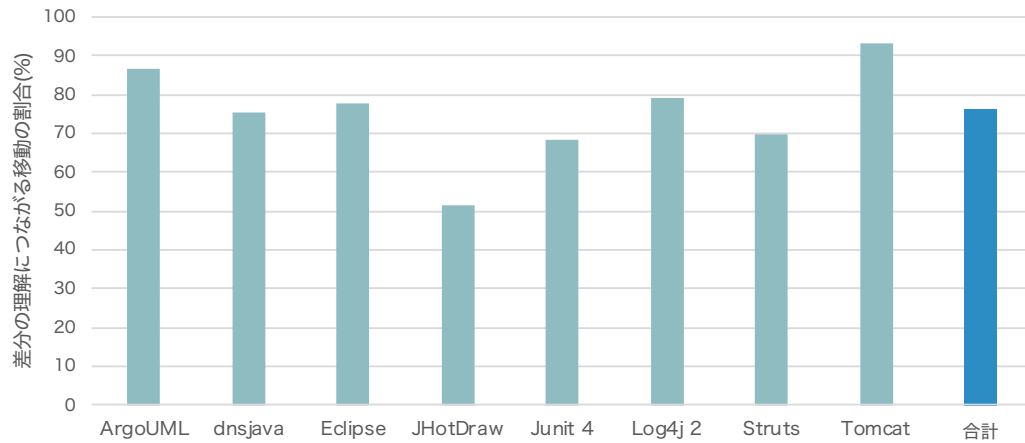
図 9 差分の理解につながる移動の割合
