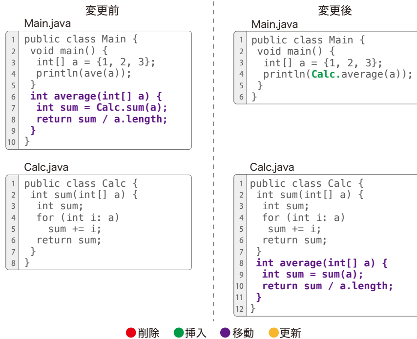
(b) 実際に行われた操作をより適切に反映する出力
