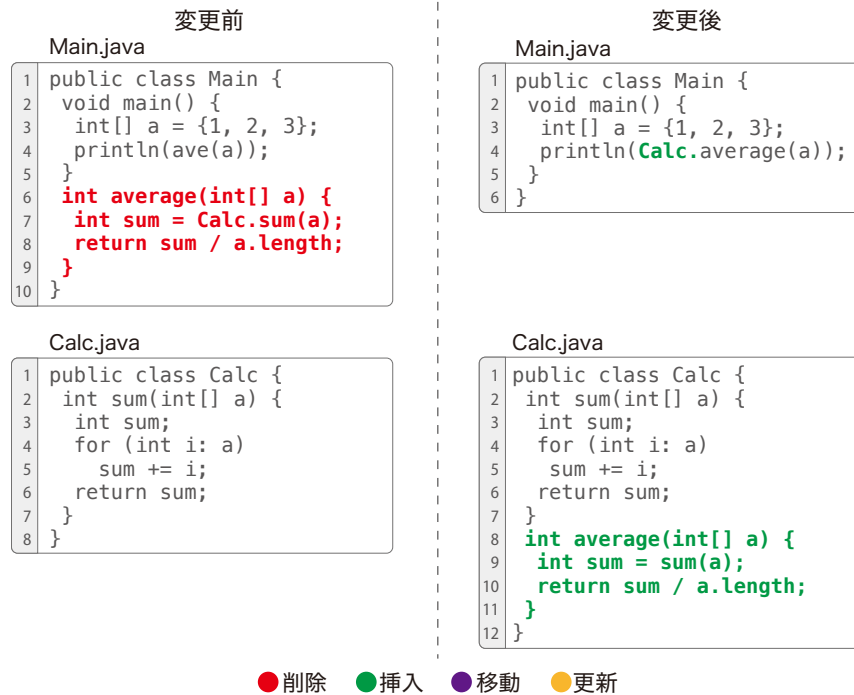
(a) GumTree の出力
