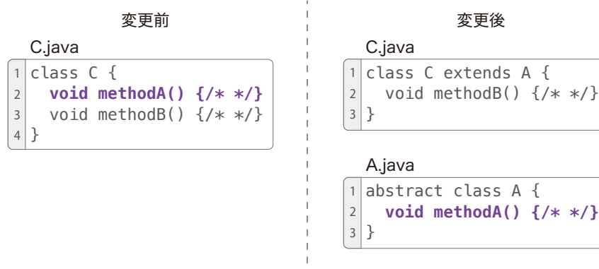
図 13 継承関係の変化のソースコードの例
