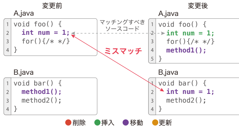
図5 不適切なマッチングによる誤検出の例
