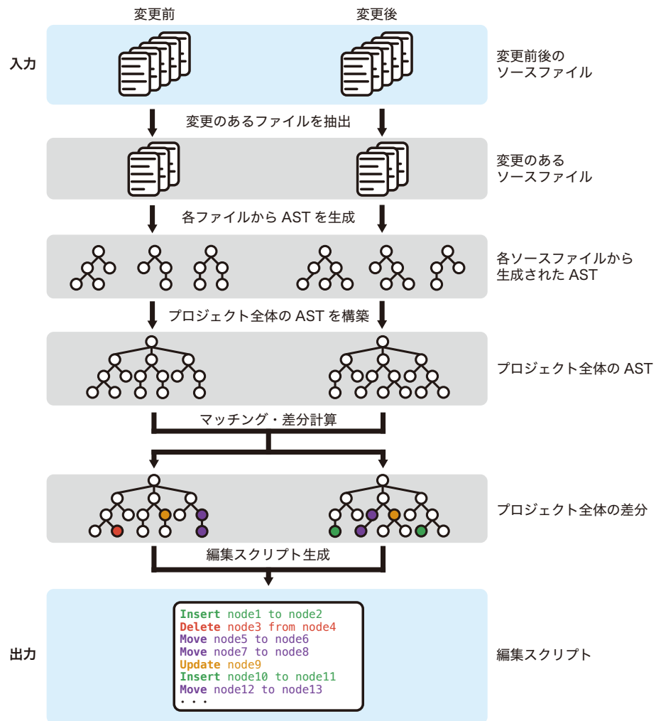
図3 提案手法の概要
