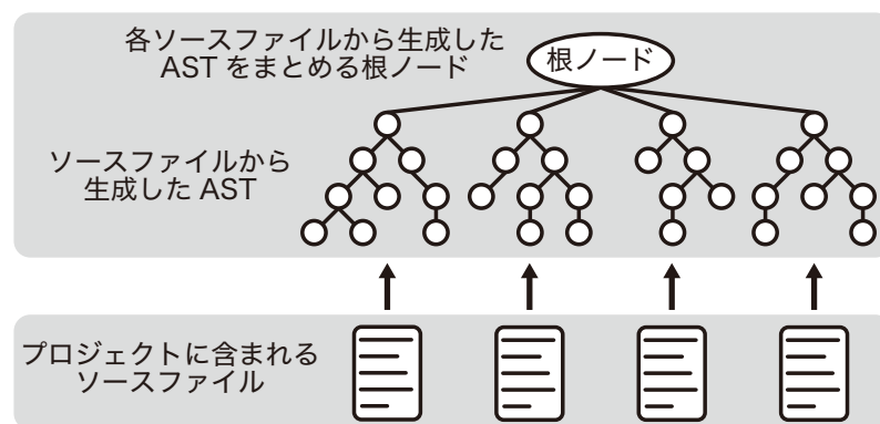
図4 プロジェクト全体の AST の構築
