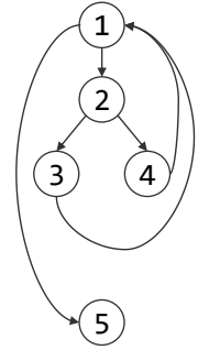
(b) 制御フローグラフ
