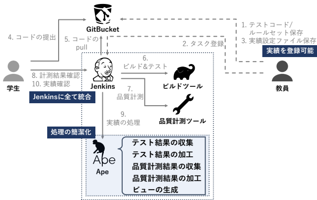
図 3 提案手法 Ape によるテストベースの教育の流れ
