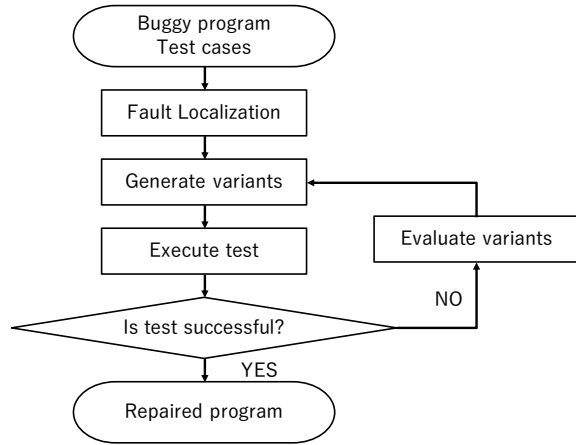
Fig. 1: Overview of GenProg
