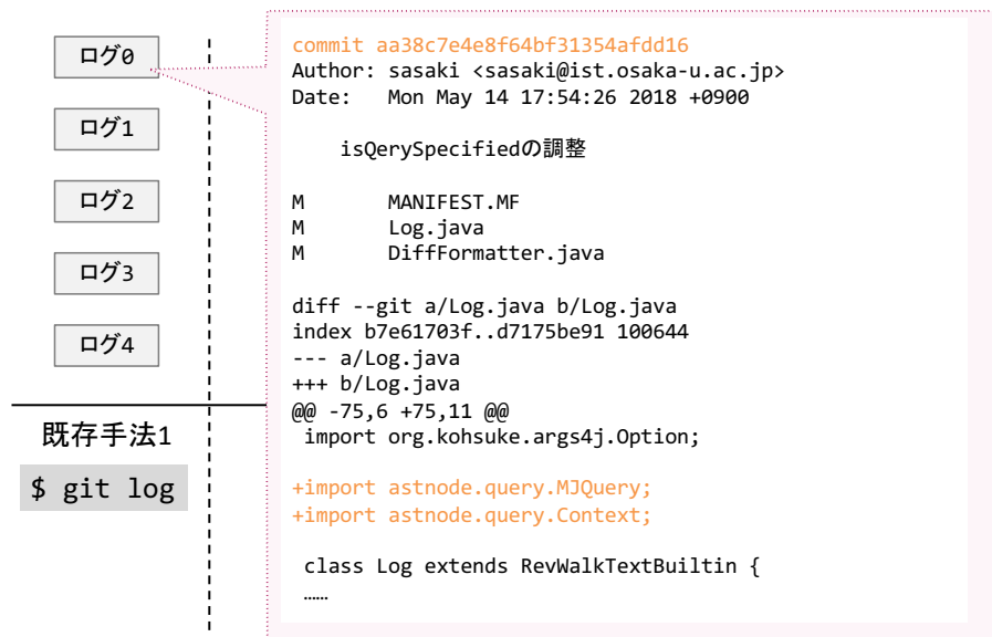
(a) あるログが持つ情報の一例
