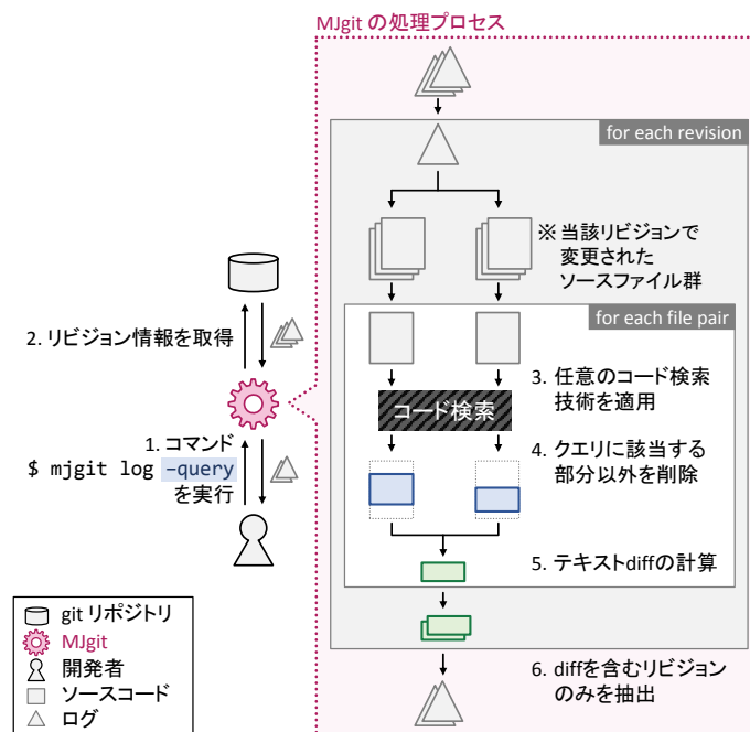
図4 MJgitにおける git-log コマンドの処理の流れ
