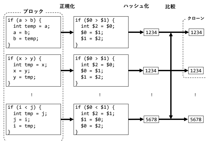
図 4 クローン検出の例
