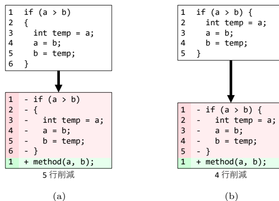
図 3 コードによって削減行数が異なる例
