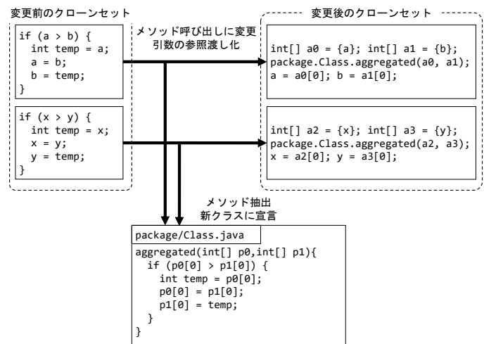
図 5 ソースコード変更の例
