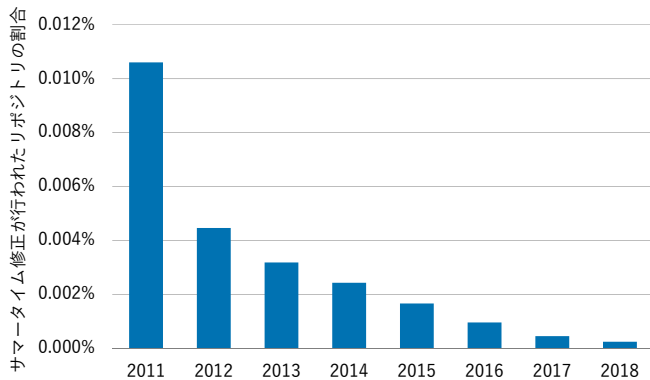
図 1 サマータイム修正が行われたリポジトリの作成時期
