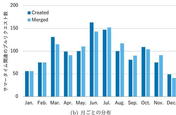
図 3 サマータイム修正時期の分布
