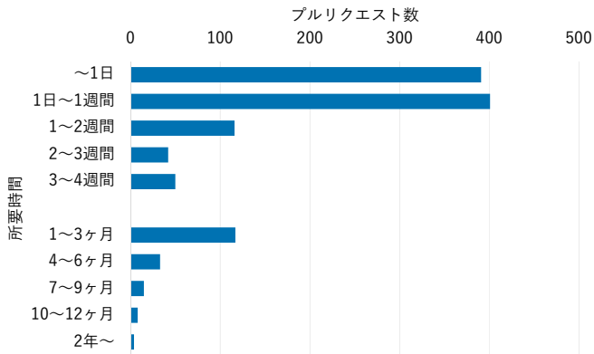
図 4 サマータイム修正が行われてからマージされるまでの所要時間
