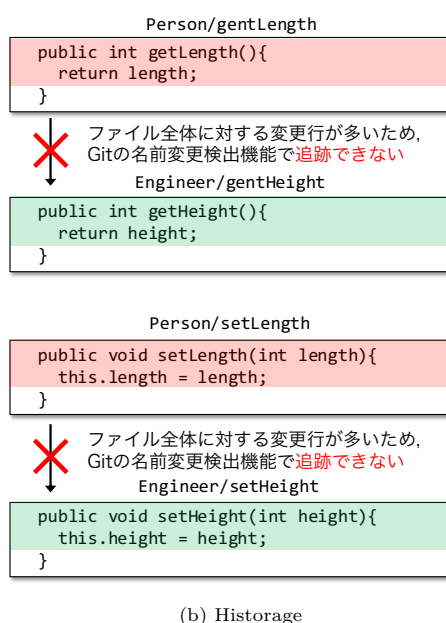
図2 Git と Historage の違い
