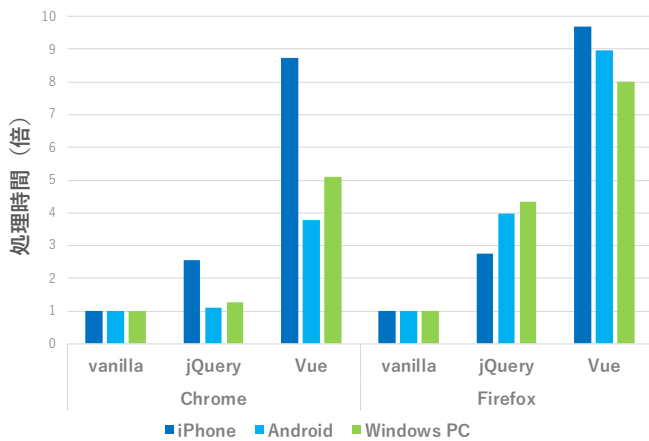
図 9: 実験結果 : DOM 要素へのクラス追加
