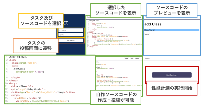
図 3: コード比較画面
