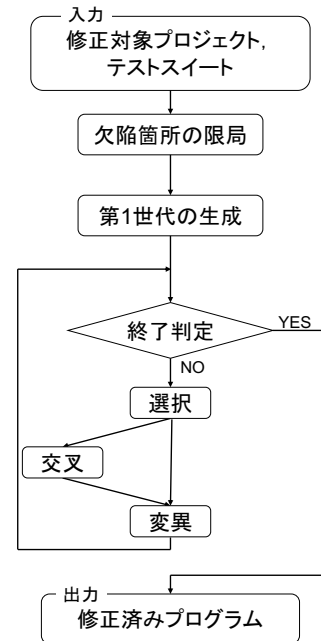
図 1: GenProg の動作の流れ
