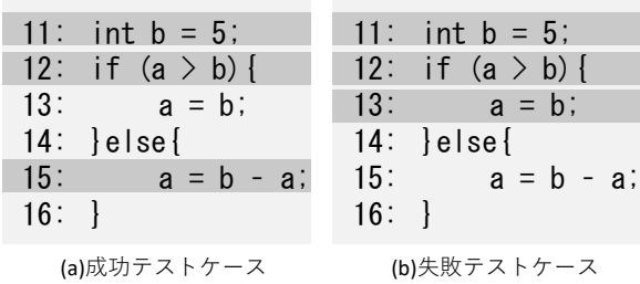
図 5 テストによるプログラムの実行経路。網掛け部分が実行されたコード。
