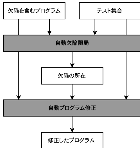
図 1 デバッグ自動化技術の概要
