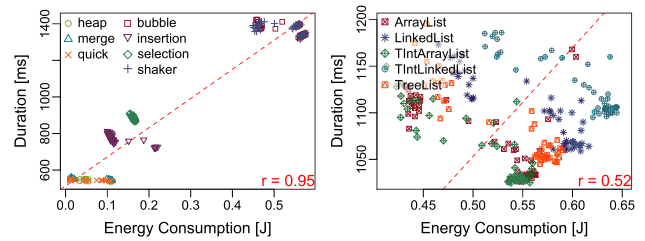
ソーティングアルゴリズム Java Collections クラス
