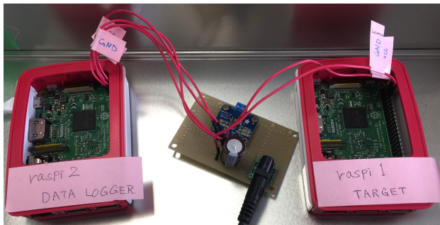
図 3 eTracker の全体図
