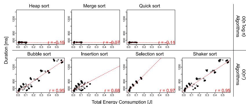
図 5 実験 1: ソーティングアルゴリズムについての詳細
