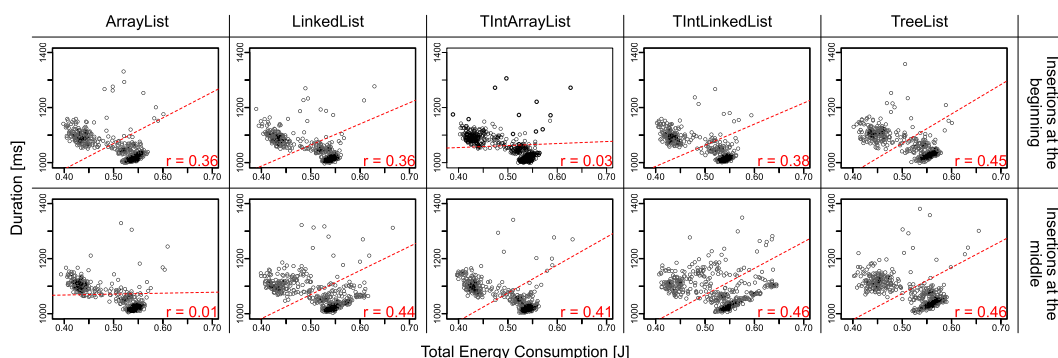
図 6 実験 1: Java Collections クラスについての詳細
