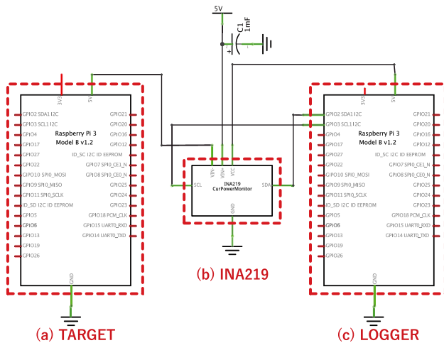
図 2 eTracker の回路図
