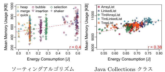
ソーティングアルゴリズム
