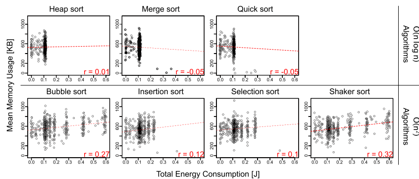
図 8 実験 2: ソーティングアルゴリズムについての詳細
