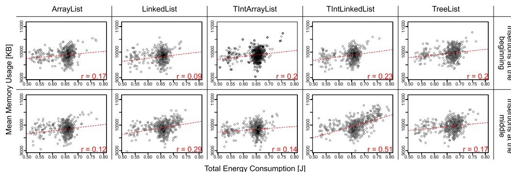
図 9 実験 2: Java Collections クラスについての詳細
