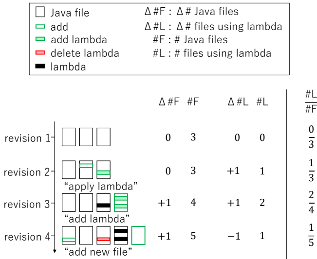
図4 リポジトリの例と調査に用いる指標の計測方法
