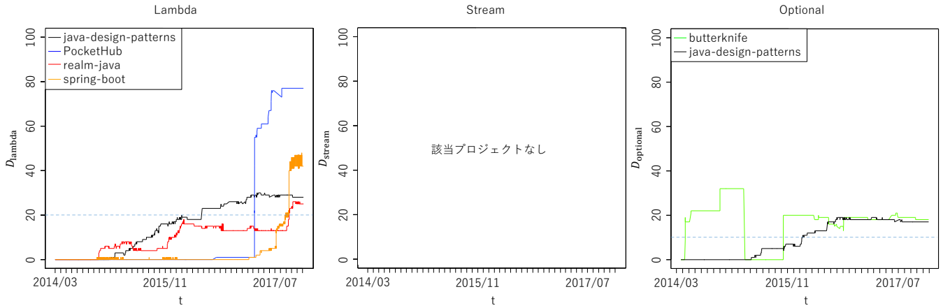
図7 「採用」とみなされたプロジェクトの各リビジョンにおける D_{\text{idiom}}
