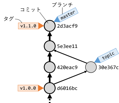
図3 コミットグラフの例
