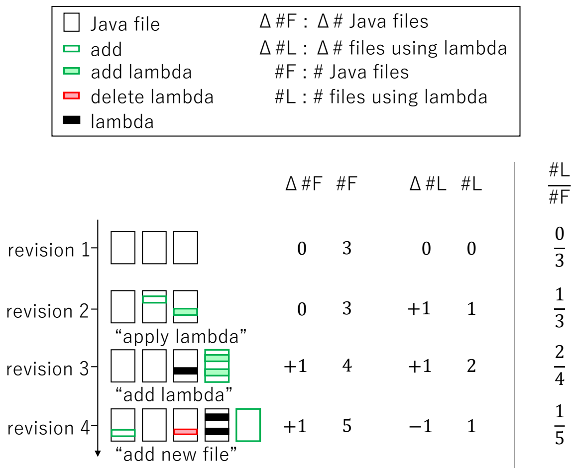
図6 リポジトリの例と調査に用いる指標の計測方法
