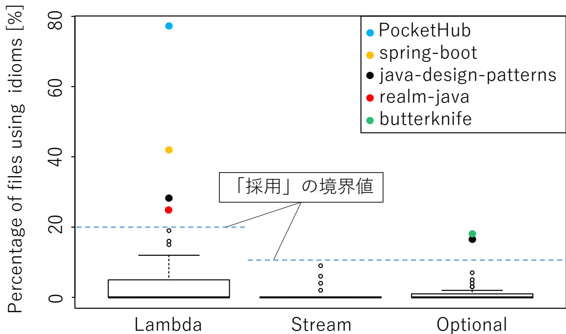
図8 最新リビジョンにおける D_{\text{idiom}} の分布
