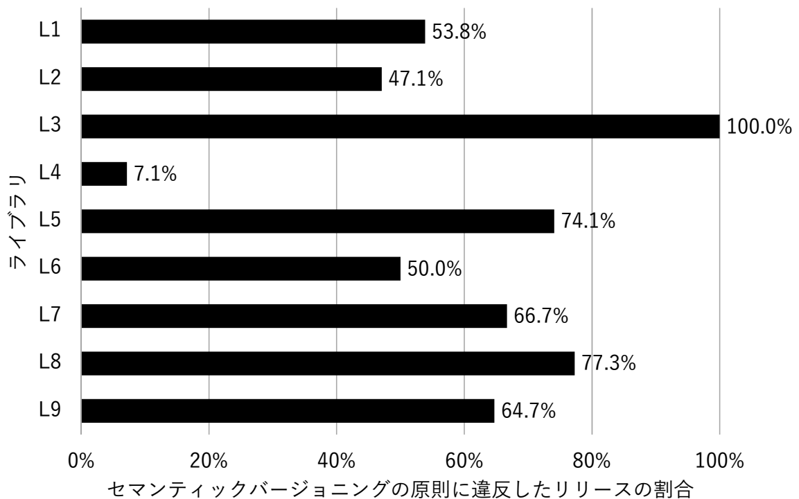
図7 セマンティックバージョニングの原則に違反したリリースの割合
