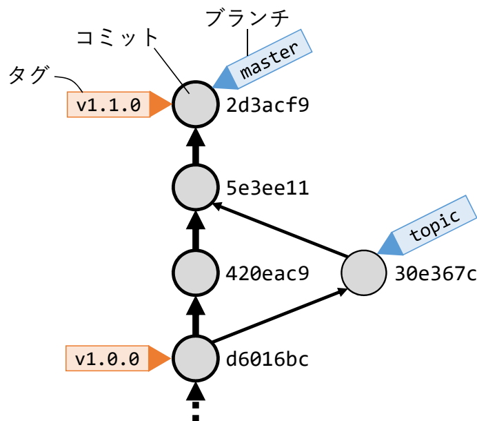
図5 コミットグラフの例
