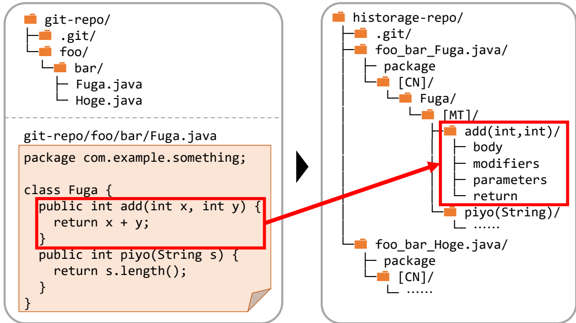
図6 Git リポジトリとそれを変換した Historage リポジトリ
