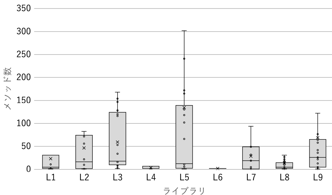
図8 本来後方互換性があるはずのリリースに含まれている後方互換性のないメソッドの数
