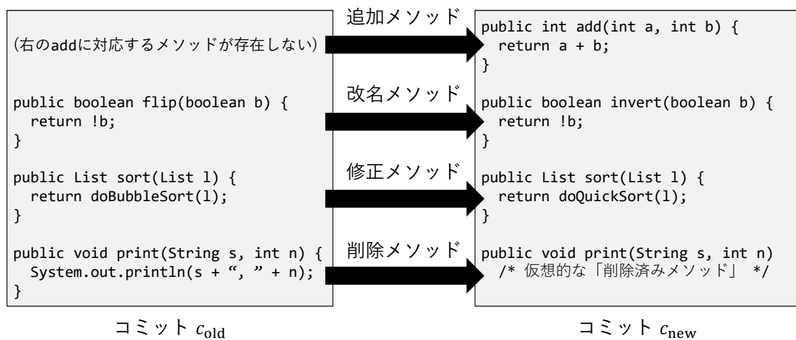
図3 メソッドの対応関係の例
