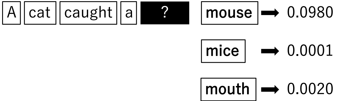
図2 言語モデルの例
