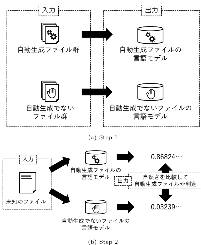
図 2 提案手法の概要
