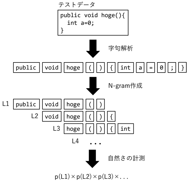
図 3 字句解析と自然さ計測の例
