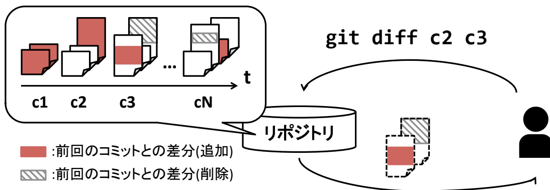
(a) 従来の Git の動作
