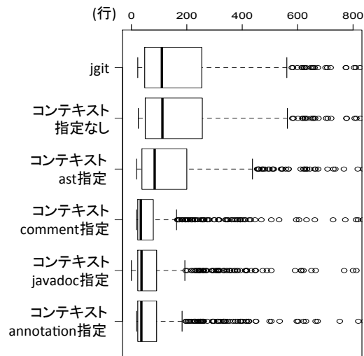
図 7: JUnit4 に対する show の出力行数
