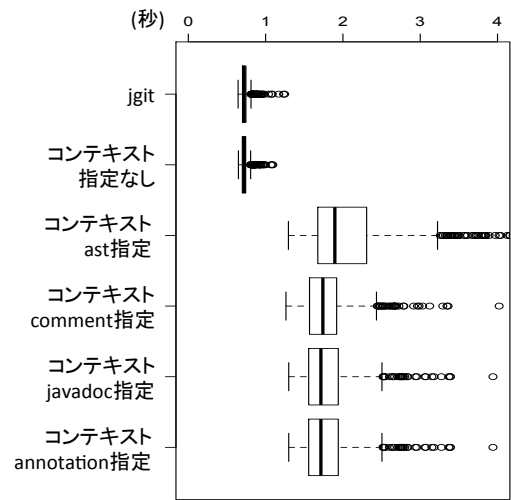
図 6: JUnit4 に対する diff の実行時間
