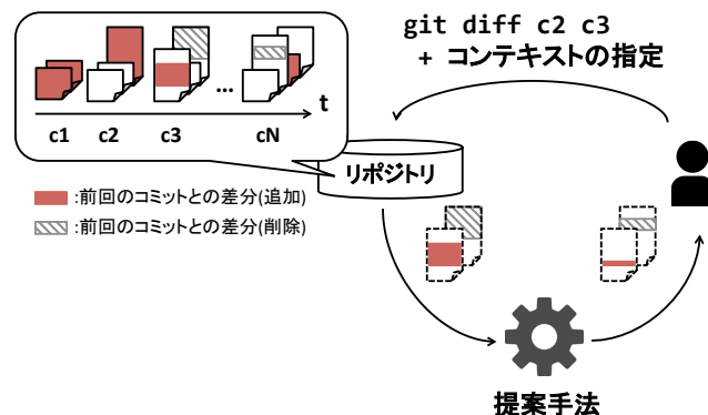
図2 提案手法の動作
