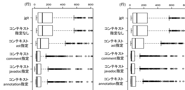
図 8 JUnit4 に対する show の出力行数
