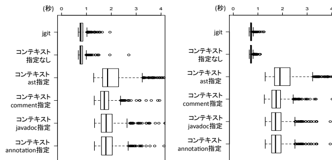
図 6 JUnit4 に対する show の実行時間
