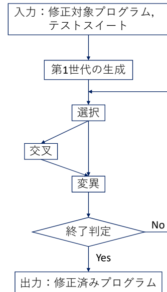
図 1 GenProg の動作の流れ
